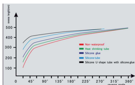
Curva inversa
